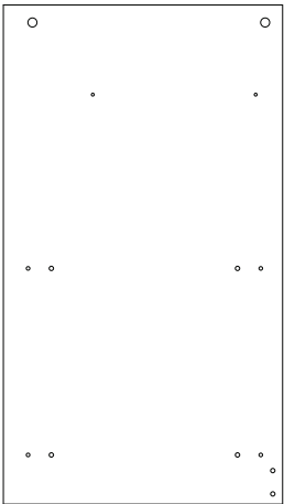
04 - 685x384x15mm - 1x
